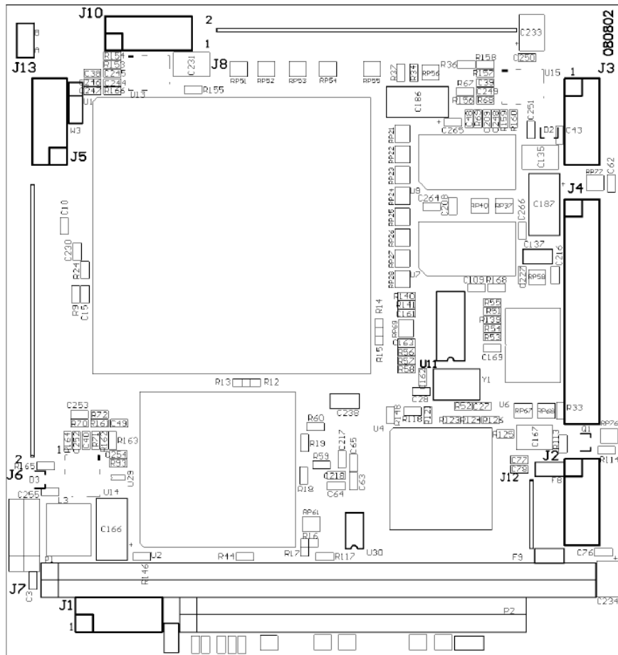
图 1-2. 连接器和跳线器的位置
