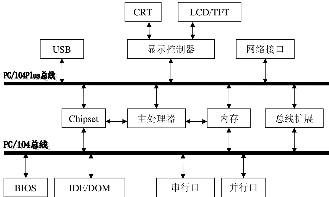
图 1-1. EM-4850 系统结构图
